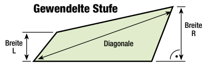
5-Eckstufe
